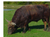
Krossbuck Kim
